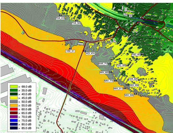
Hluková mapa: současný stav bez protihlukové stěny – výhledový rok 2030
