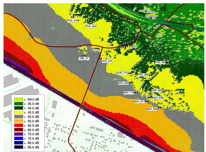
Varianta 7 - Pohltivá protihluková stěna výšky 5m, délka 600m (maximální varianta)
